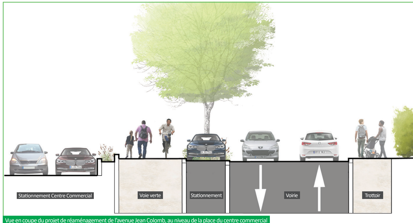
Vue en coupe du projet de réaménagement de l'avenue Jean Colomb, au niveau de la place du centre commercial
